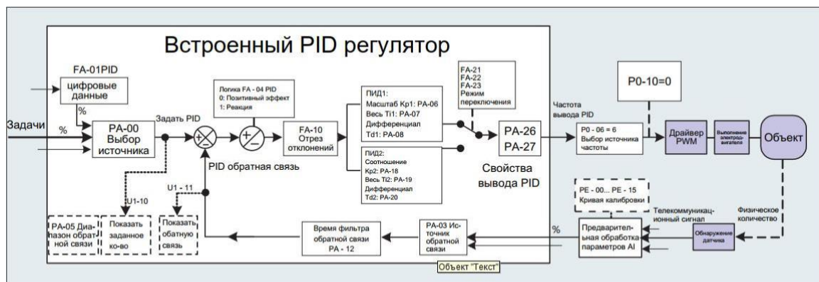
Рисунок 4 - 19 Принцип управления замкнутым циклом частот
