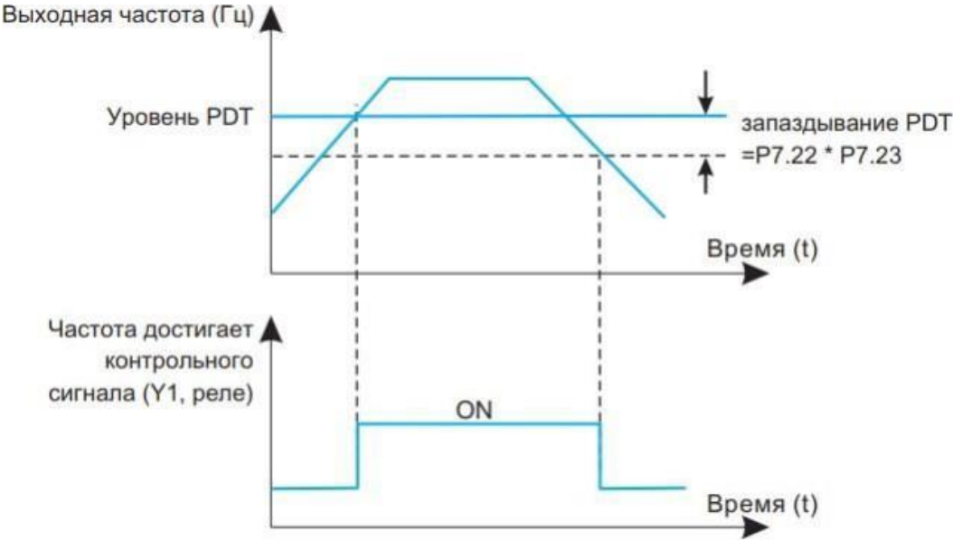
Рисунок 6 - 15 Уровень PDT
