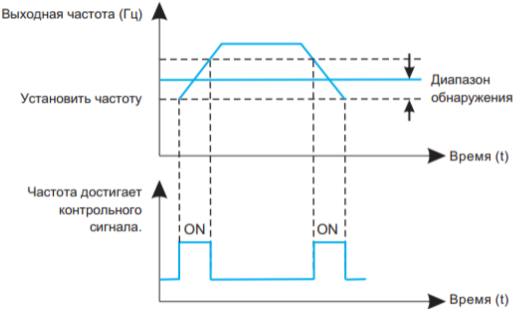
Рисунок 6 - 16 Диаграмма диапазона обнаружения прихода частоты
