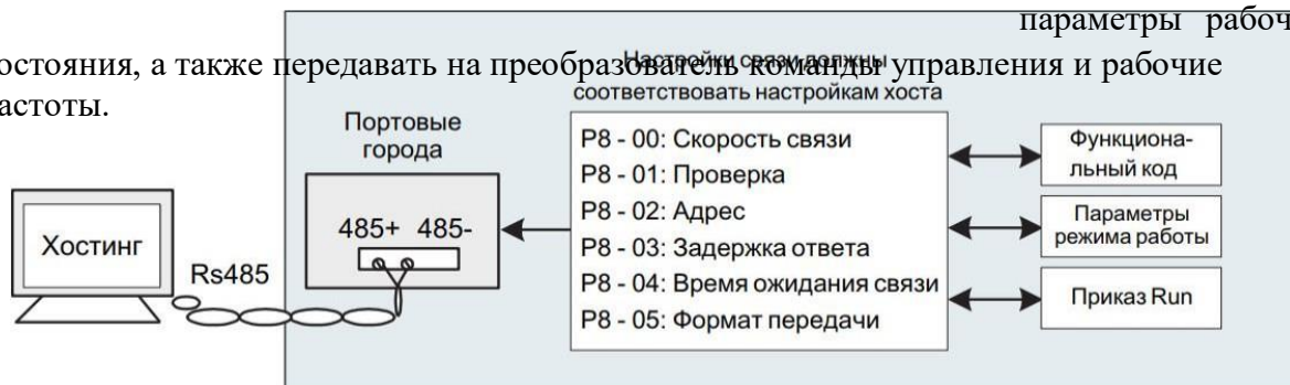
Рисунок 4 - 30 Параметры связи
