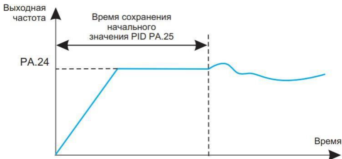
Рисунок 6 - 25 Функциональная схема начального значения PID
