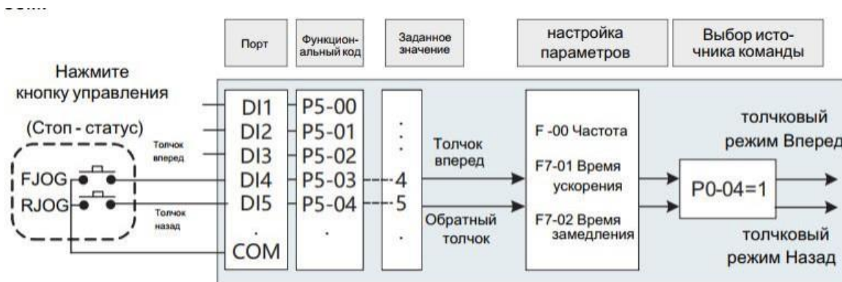
Рисунок 4 - 16 Настройка параметров точечного движения в режиме DI
