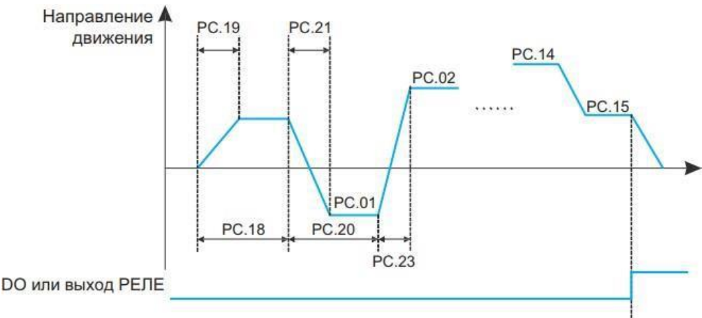
Рисунок 6 - 29 Простая схема PLC
